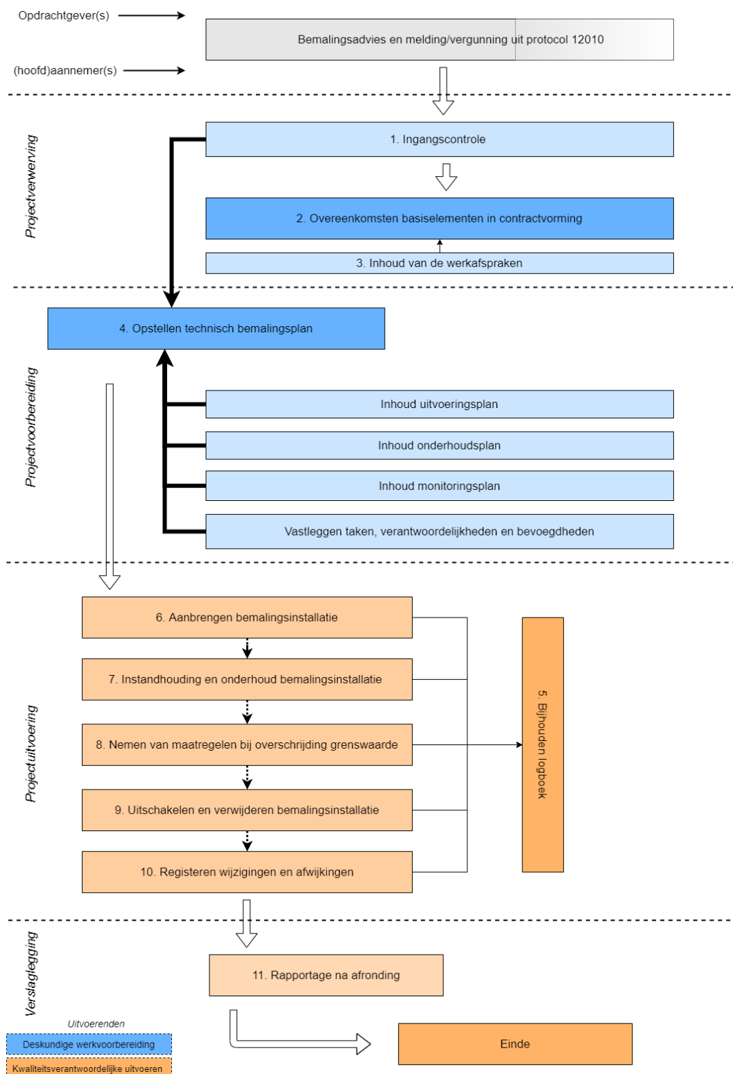
Figuur 1. Stroomschema 'Werkvoorbereiding en uitvoering bemaling'. Cat.1 en Cat.2 bemalingen.
