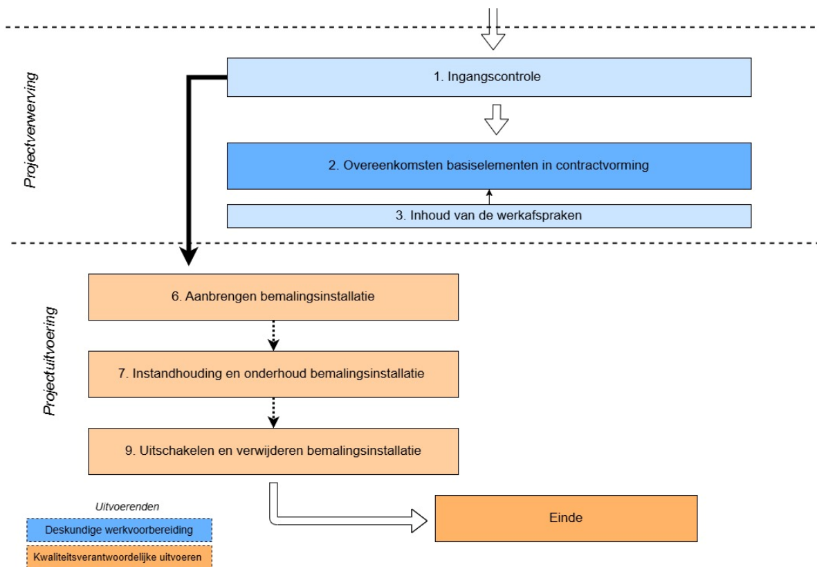
Figuur 2. Stroomschema ‘Werkvoorbereiding en uitvoering bemaling’. Cat.3 bemalingen.
